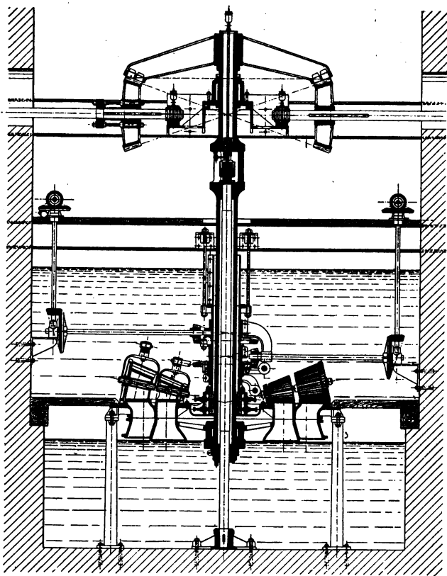
Fig. 51. Girard-Turbine von Anreva & Co. in Erfurt.
